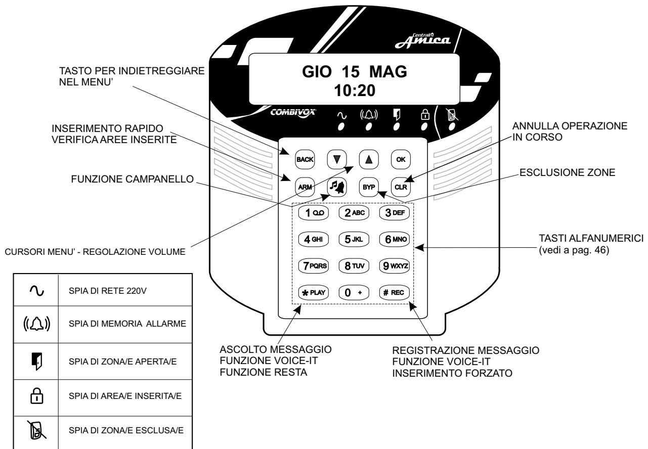
Figura 2 : riepilogo tasti e indicazioni luminose della tastiera (vedi a pag. 45).
