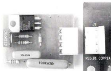
Fig. 8 - REGOLATORE DI COPPIA - TORQUE ADJUSTMENT CARD - RÉGULATEUR DE COUPLE
