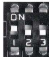
Fig. 9 - DIP DI SELEZIONE PROGRAMMA - PROGRAMME SELECTION DIP - DIP DE SELECTION PROGRAMME
